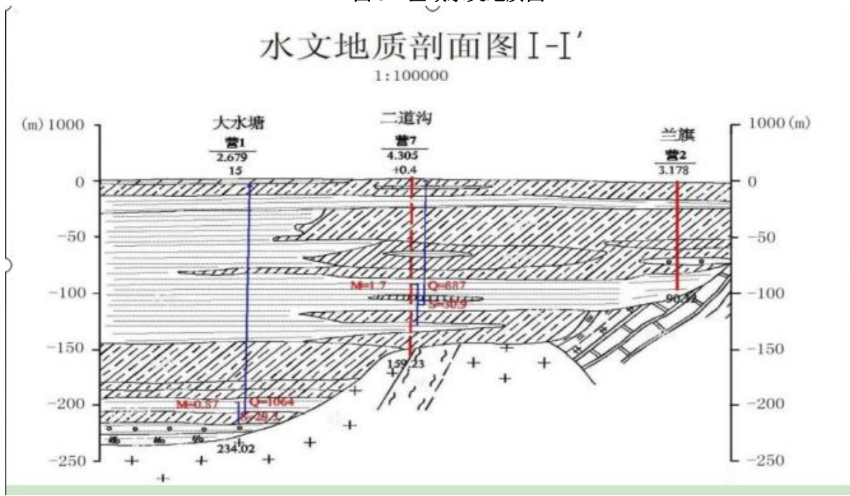
图 3-2 水文地质剖面图
