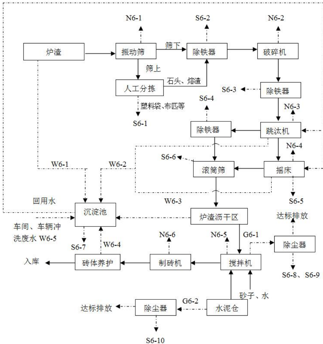
图 4-5 炉渣制砖工艺流程图
