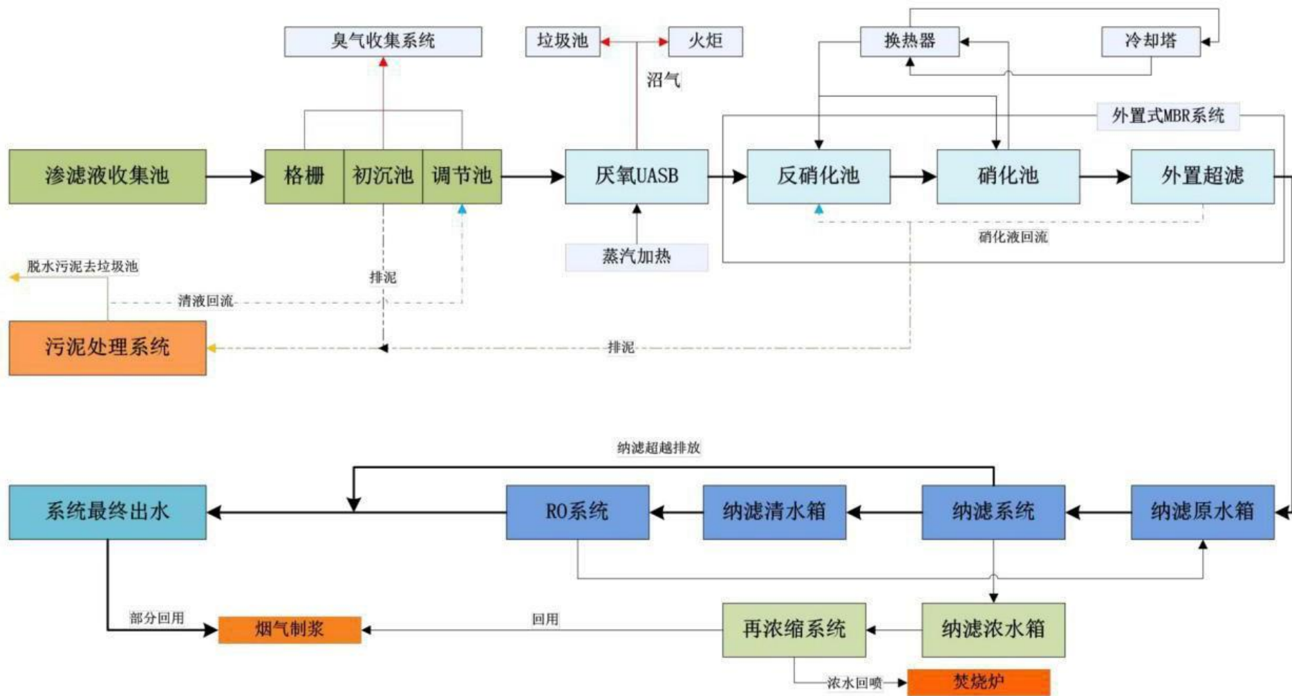
图 2.4-1 渗滤液处理工艺流程图
