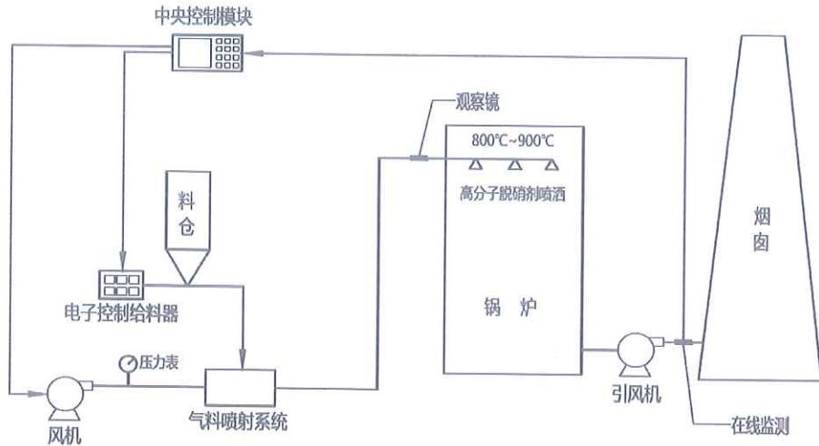
图 2.4-2 PNCr 工艺流程图
