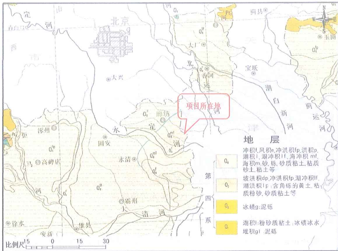
图 2.2-1 地形地貌图
