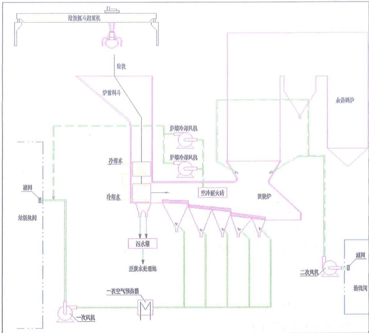
图 2.4-1 焚烧系统流程图
